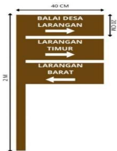
Gambar 1. Desain Plang
